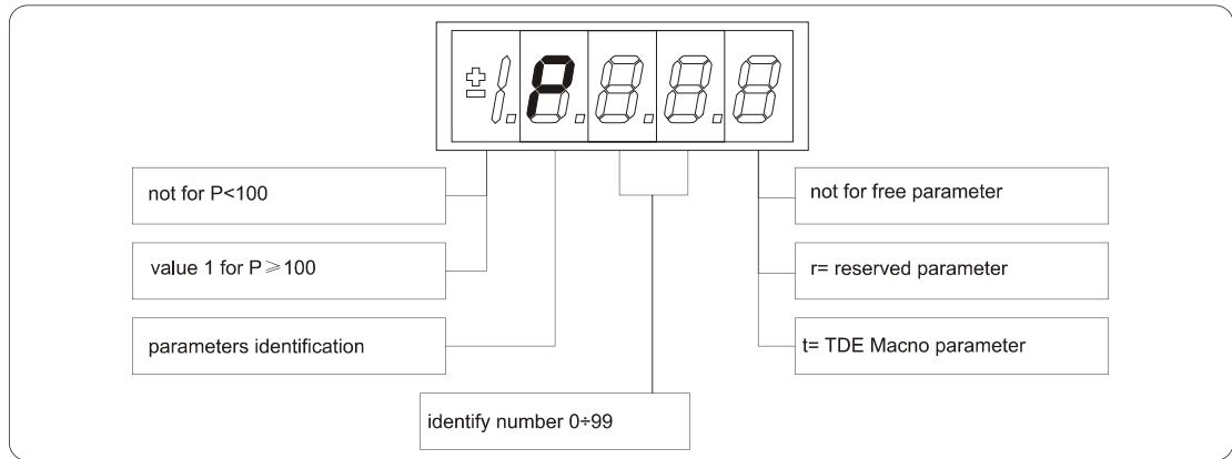
FIG. 2 (Parameters PAR)
